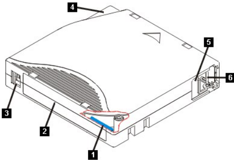
图 14. LTO Ultrium 1500 GB 数据盒带
