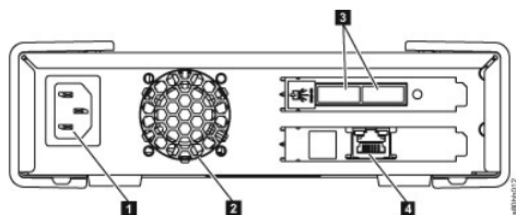
图 5. 外置 SAS 磁带机的后面板
