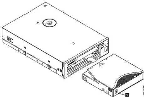
图 15 装入盒带
