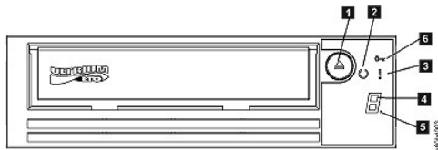
图 3. 前面板
