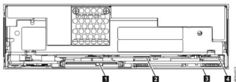
图 4. 内置 SAS 磁带机的后面板
