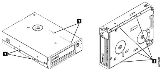
图 8. 磁带机上的安装孔
