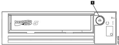
图 13. 重置磁带机
